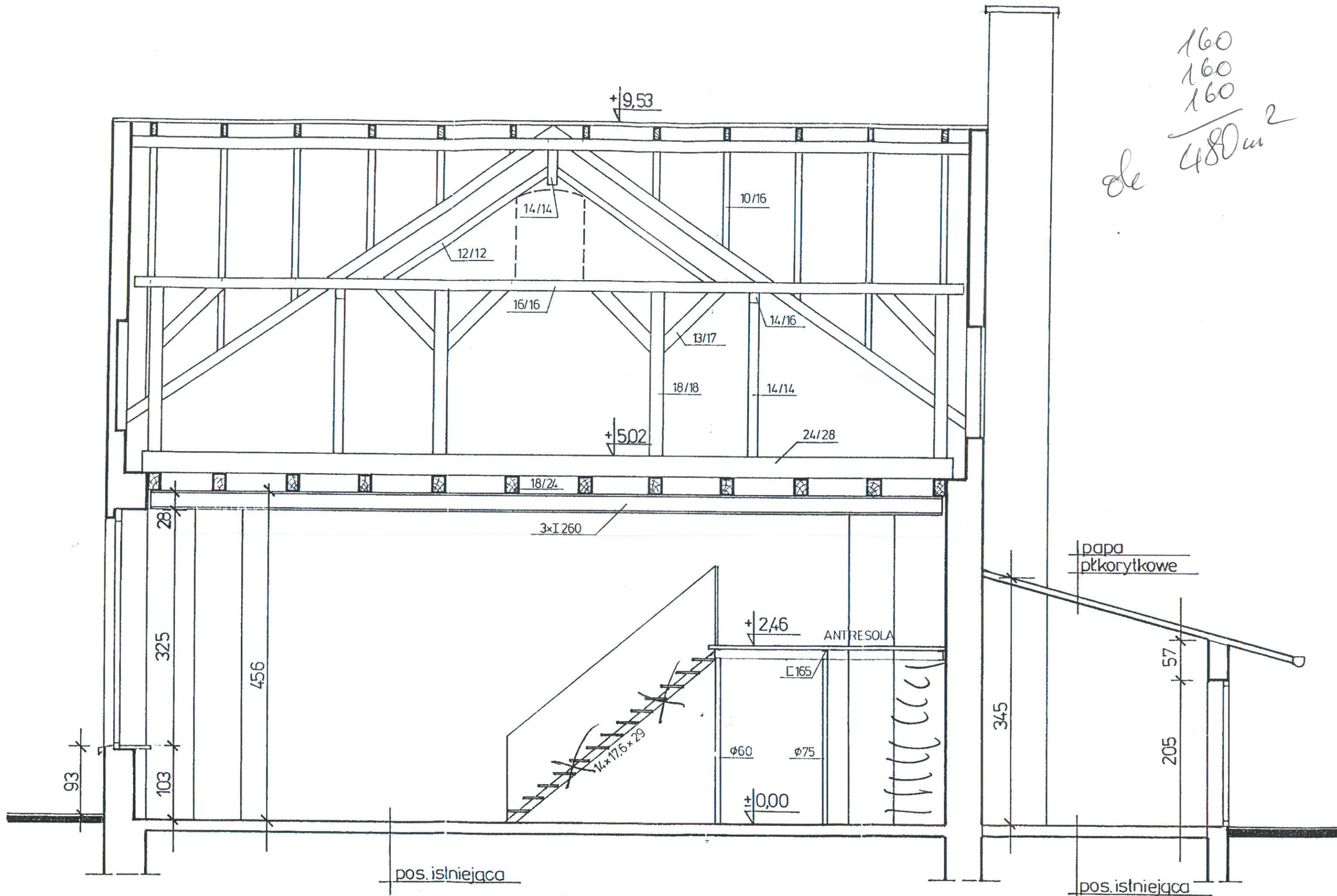
PRZEKRÓJ I-I 1:50
